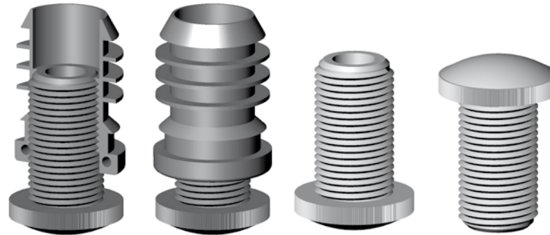
Verstellgleiter für Rundrohr, Rändelschraube M16x30 mit gewölbter Stellfläche Height adjuster for round tube, screw M16x30 with knurled vaulted base Insert-vérin pour tube cylindrique, vis M16x30 avec embase moletée bombée
